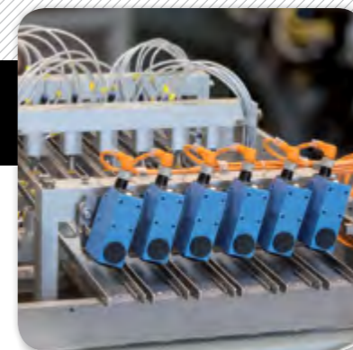
2. Fotocèl·lula.
